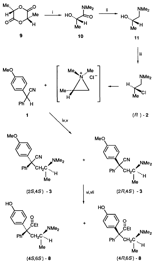
Scheme 2 Reagents: i, \text{Me}_2\text{NH} ; ii, LAH; iii, \text{SOCl}_2 ; iv, \text{LiNPr}^+_2 ; v, chromatography; vi, \text{EtMgBr} ; vii, \text{BBr}_3
